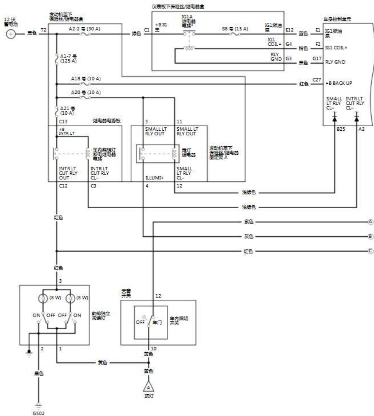
车内照明灯电路图
